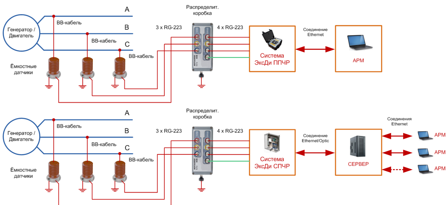
Типовые функциональные блок-схемы диагностики состояния изоляции генераторов/двигателей методом выявления частичных разрядов с использованием ёмкостных датчиков ТСС 24
